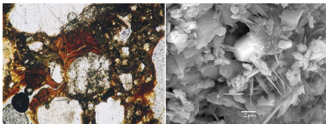
Αργιλικές επικαλύψεις σε ένα Rhodoxeralf (πολωτικό μικροσκόπιο) (αριστερά) και ορυκτά του “σμεκτίτη” (ηλεκτρονικό μικροσκόπιο) (δεξιά).
